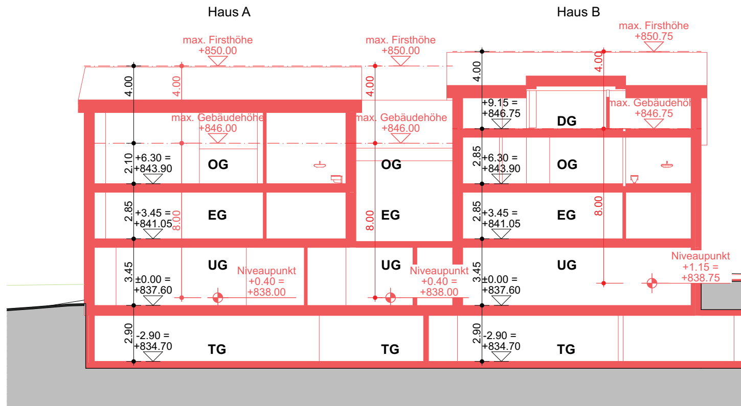
Schnitt A (Längsschnitt)
