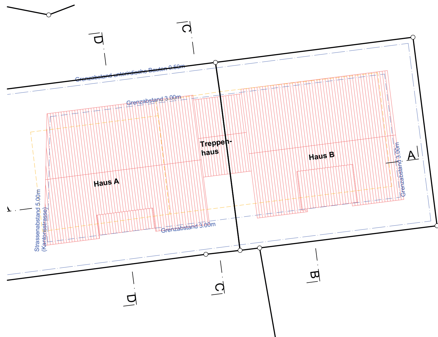
Dachaufsicht
