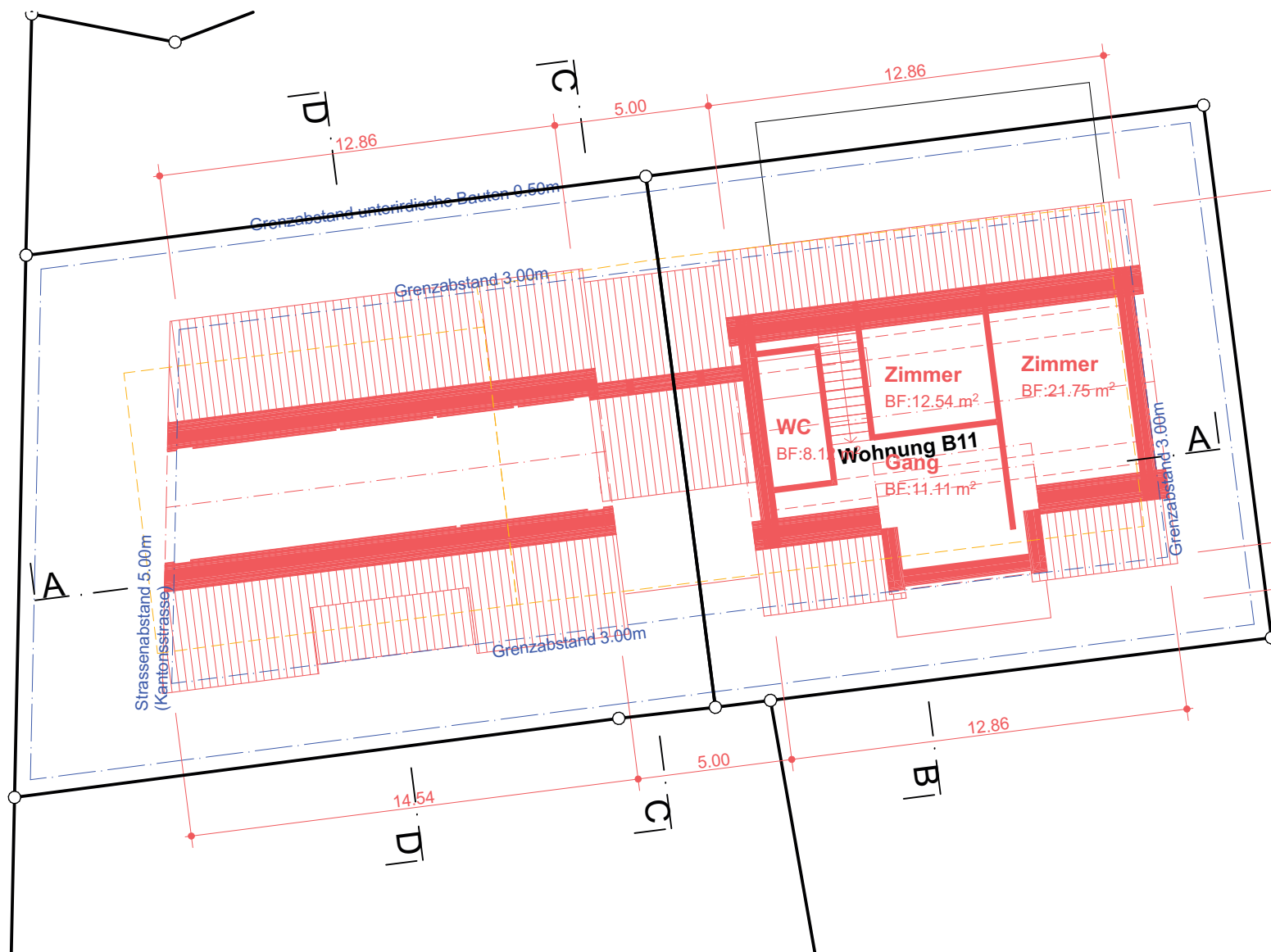
Dachgeschoss
