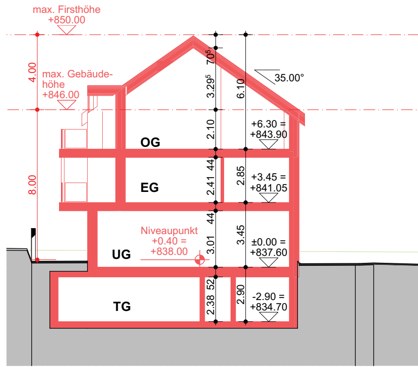
Schnitt D (Haus A)
