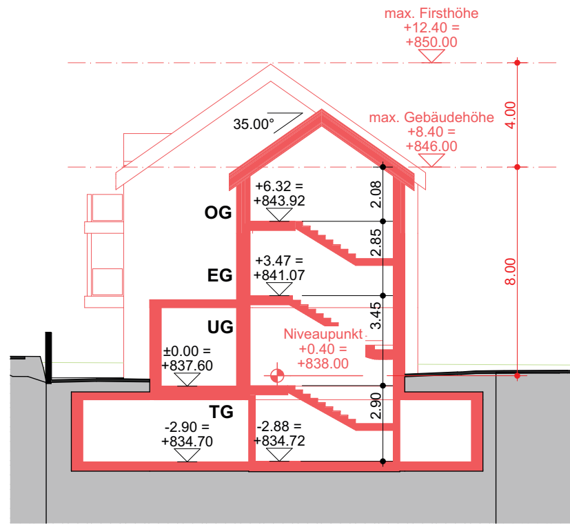
Schnitt C (Treppenhaus)
