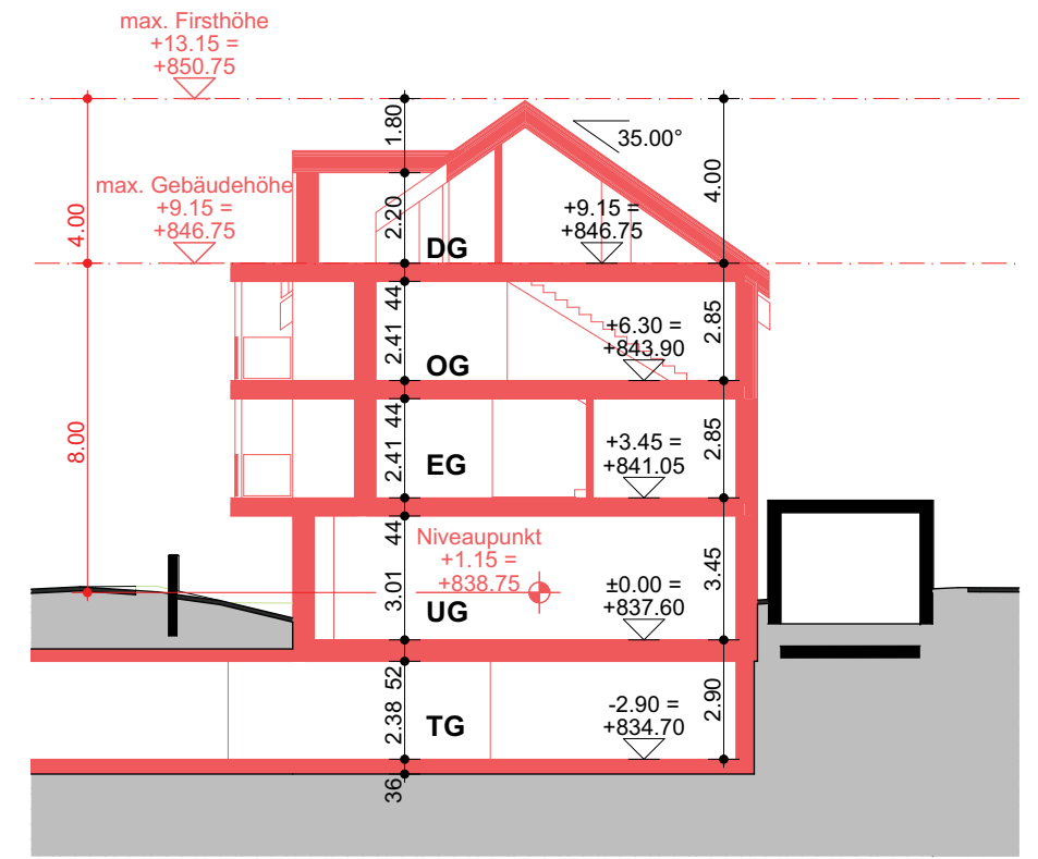
Schnitt B (Haus B)
