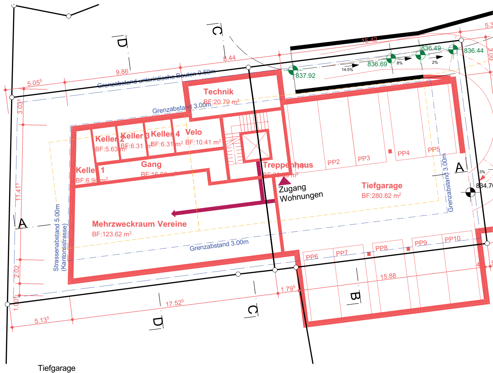
Untergeschoss
